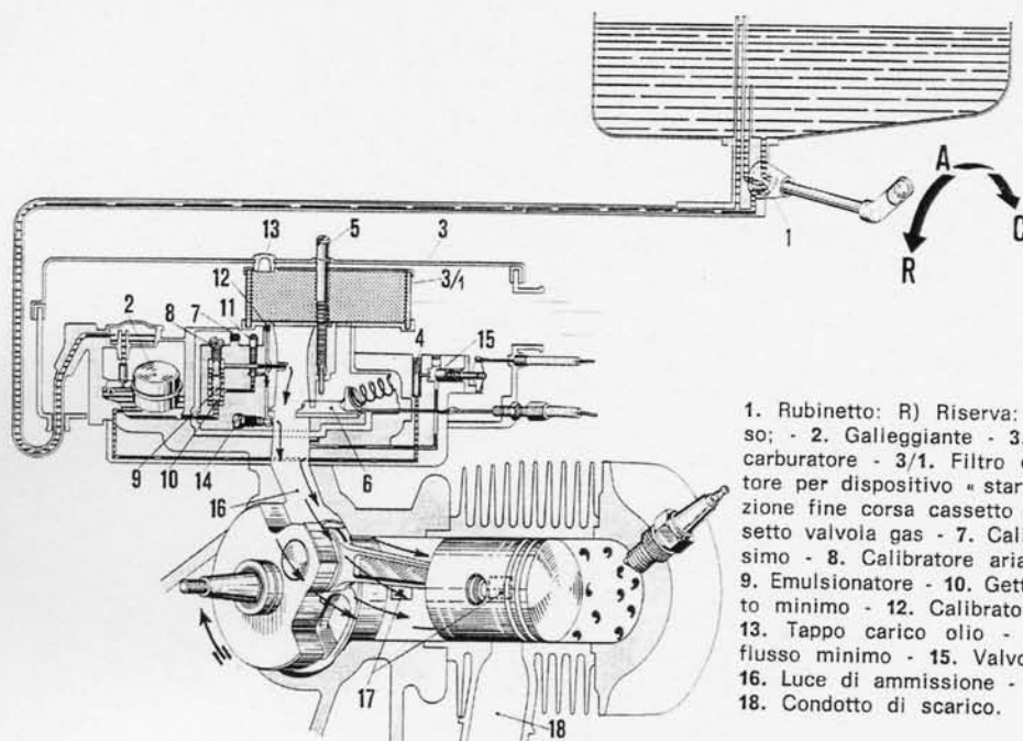
Schema dell'alimentazione e distribuzione
